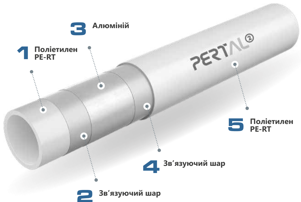
Конструкція труби PERTAL 2
